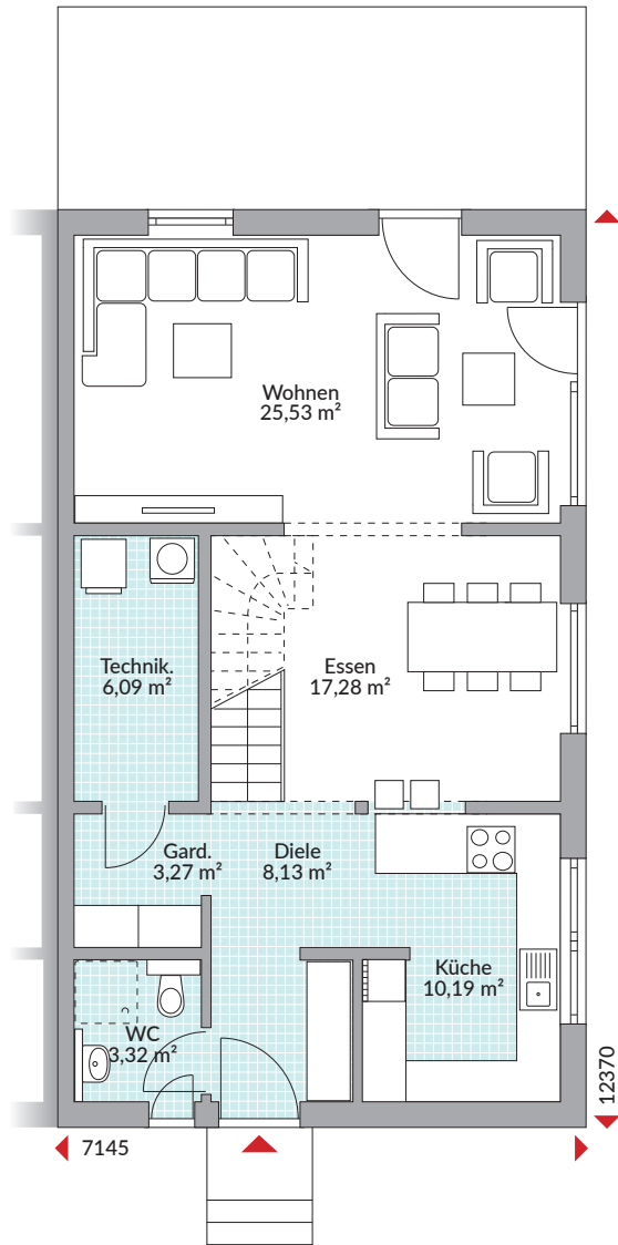
Erdgeschoss 73,81 m 2
