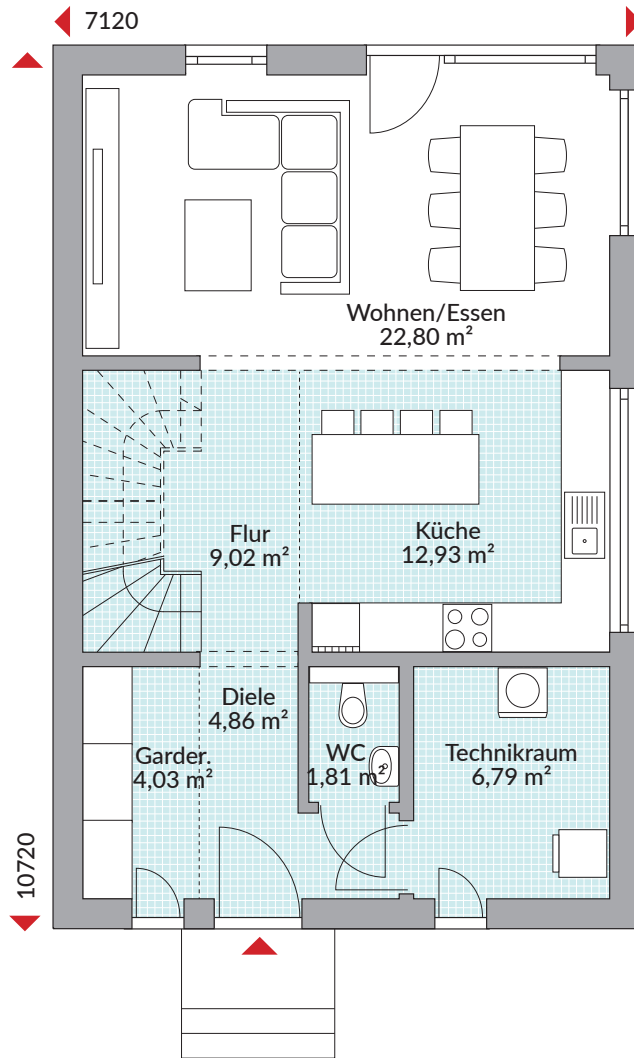
Erdgeschoss 62,24 m 2
