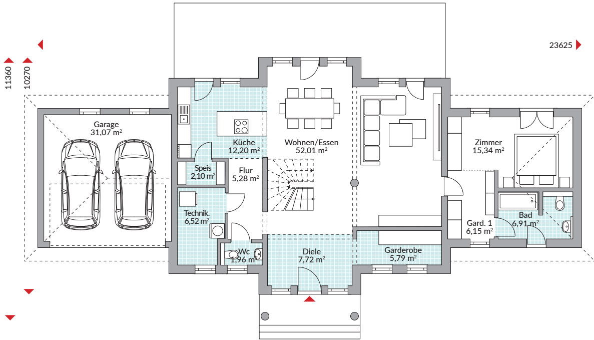
Erdgeschoss 153,05 m 2
