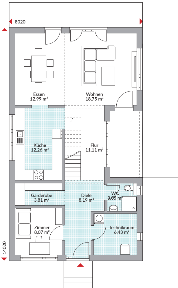
Erdgeschoss 84,66 m 2
